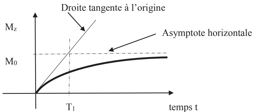
Figure 2 – Relaxation longitudinale
