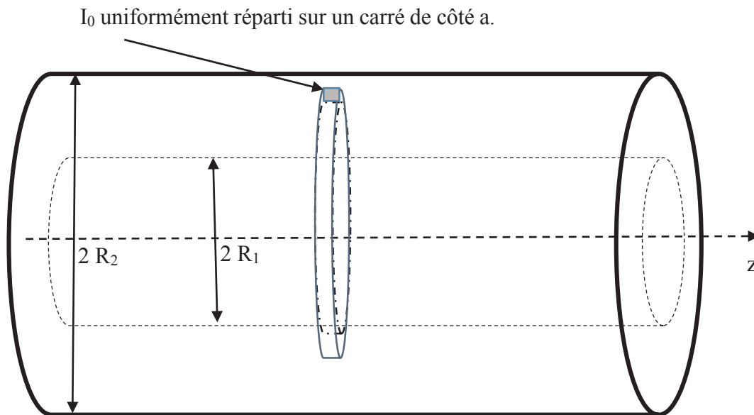
Figure 6 – Solénoïde épais
