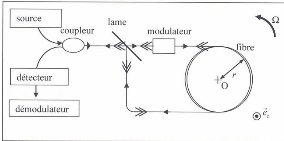
Figure 5 - Interféromètre de Sagnac à fibre optique
