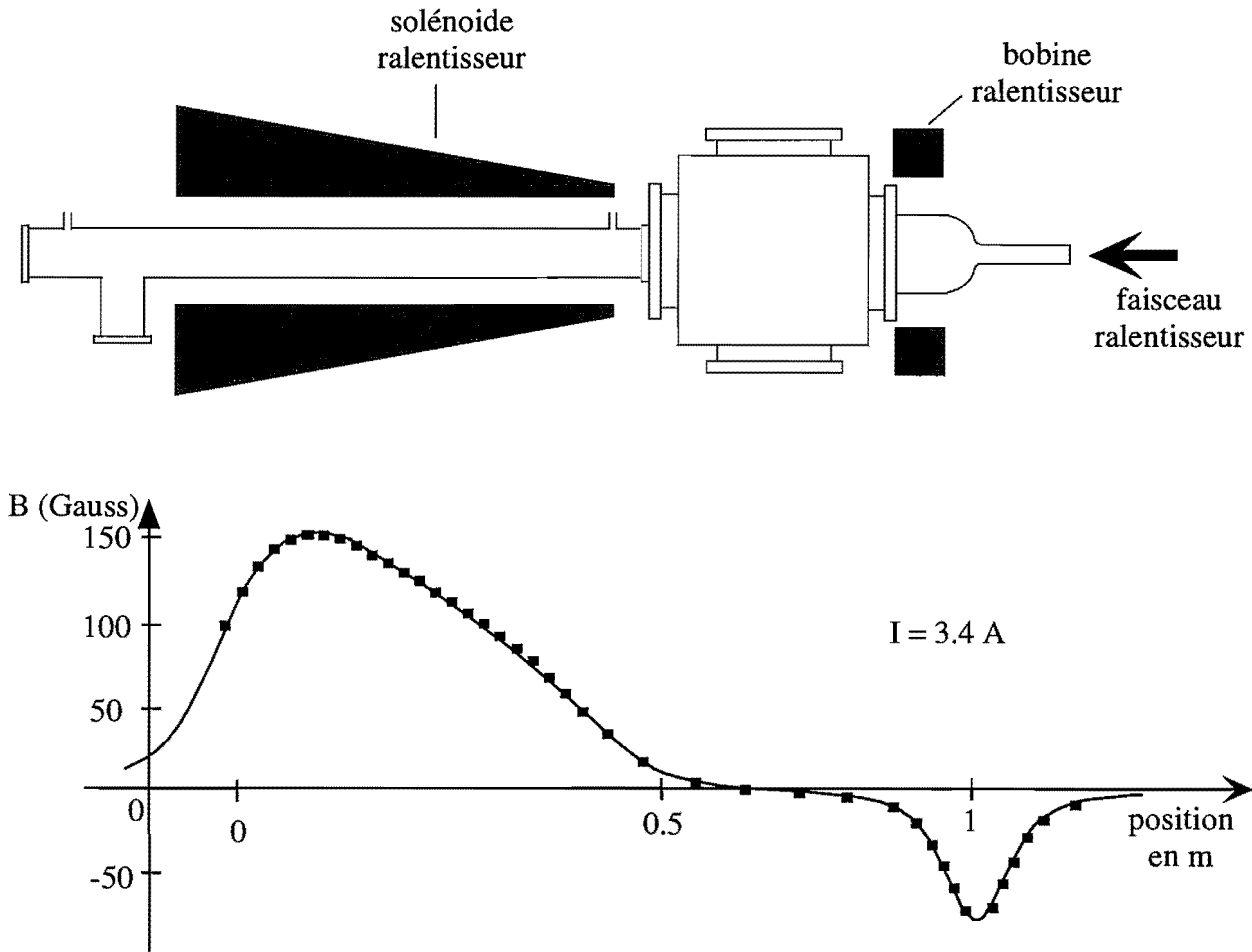
Figure 3 Les deux enroulements du ralentisseur (en noir sur le schéma du haut) sont parcourus par un courant I = 3,4 \text{ A} . La composante B_z du champ magnétique sur l'axe, exprimée en gauss ( 1 \text{ Gauss} = 10^{-4} \text{ T} ) est représentée en fonction de z (les carrés correspondent aux mesures directes du champ et la courbe en trait plein au champ calculé).
