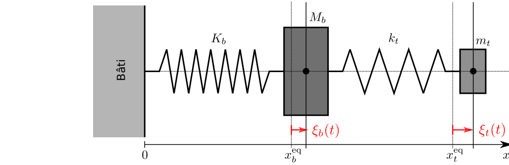
FIGURE 4 – Haut : schéma de principe du détecteur Explorer (source : adapté du site http://www.lnf.infn.it/esperimenti/rog ). Bas : modélisation de la barre d'aluminium muni du transducteur par deux oscillateurs mécaniques de masses M_b et m_t couplés par des ressorts de raideur K_b et k_t , avec M_b \gg m_t . Les deux oscillateurs sont accordés sur la même fréquence de résonance. Les positions d'équilibre des masses M_b et m_t sont respectivement x_b^{\text{eq}} et x_t^{\text{eq}} .
