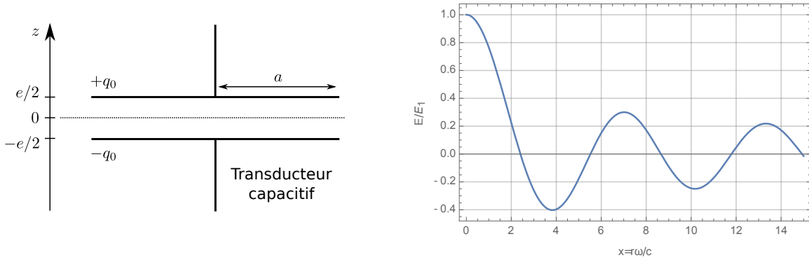
FIGURE 6 – Gauche : schéma de principe du transducteur capacitif dont les armatures sont espacées d'une distance e(t) . Droite : allure de la fonction E(x)/E_1 .
