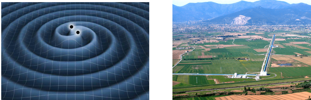
FIGURE 1 – Gauche : illustration représentant les ondes gravitationnelles générées par deux trous noirs orbitant l'un autour de l'autre et se propageant dans l'espace. Droite : détecteur interférométrique européen Virgo situé près de Pise en Italie.
