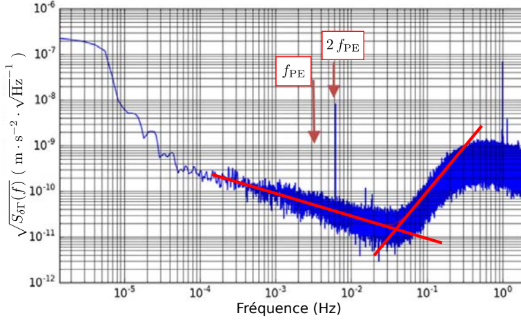
FIGURE 4.1 – Densité spectrale de puissance \sqrt{S_{\delta\Gamma}} de la différence des accélérations \delta\Gamma appliquées aux deux masses de test. La fréquence f_{\text{PE}} à laquelle l'oscillation signalant une violation du principe d'équivalence est attendue est indiquée sur le graphe. Les deux lignes correspondent à des ajustements par une loi de la forme y = af^\alpha .
