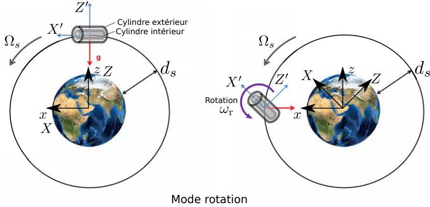
FIGURE 2.2 – Mode d'opération rotation du satellite MICROSCOPE : le satellite tourne sur lui-même, autour de l'axe (O_s y') à la pulsation \omega_r . Comme précédemment, la position du satellite est repérée à tout instant par l'angle \theta_s . À gauche \theta_s(t) = -\pi/2 , à droite \theta_s(t' > t) = 0 .
