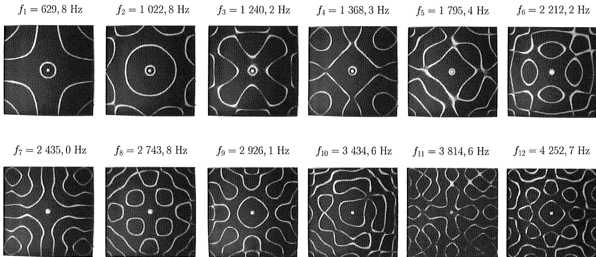
FIGURE 4 – Figures de Chladni observées avec la plaque d'épaisseur h_1 = 1 \text{ mm} . Pour chaque mode de résonance (un motif spatial), on précise la fréquence f_i associée, avec i = 1, \dots, 12 . Source : The Journal of the Acoustical Society of America 137 (2015).
